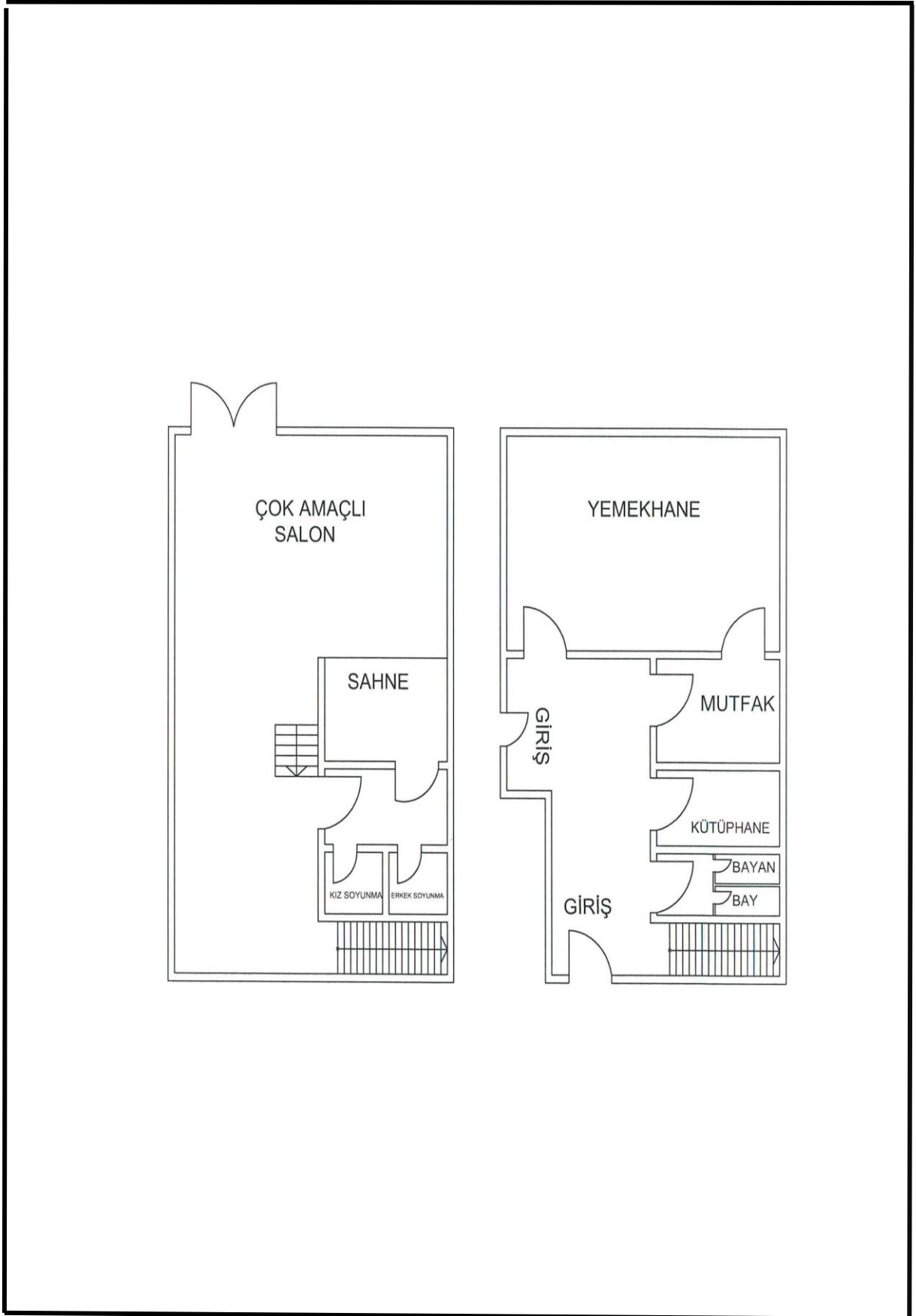
Şekil 7: Okul Ek Bina Yerleşim Planı
